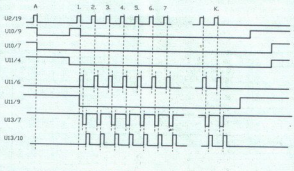
Slika 2B. Potek signalov ob selektiranju.
